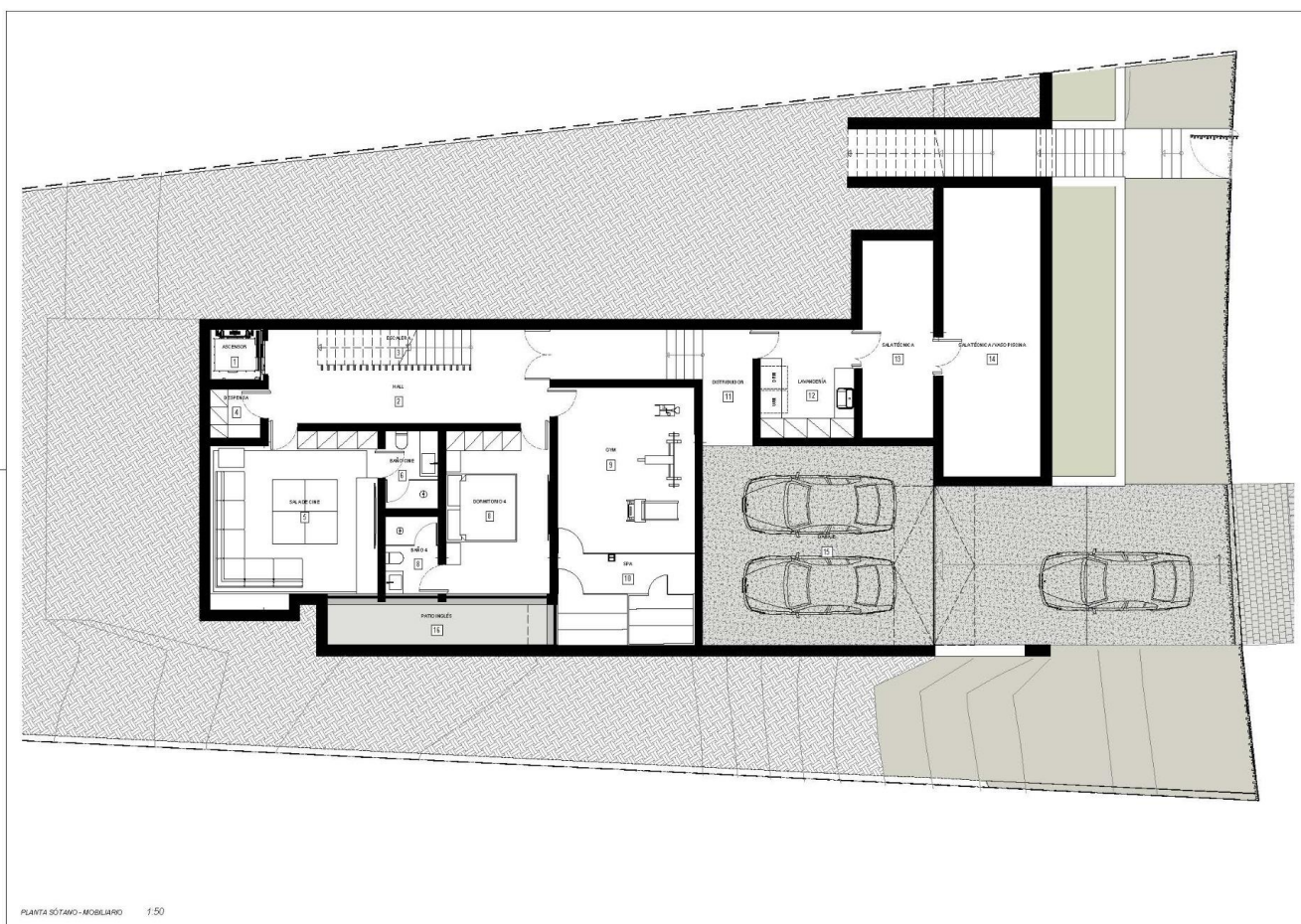
PLANTA SOTANO-MOBILIARO 1/50
