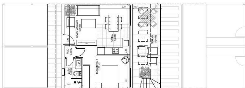
PLANTA SEGUNDA
