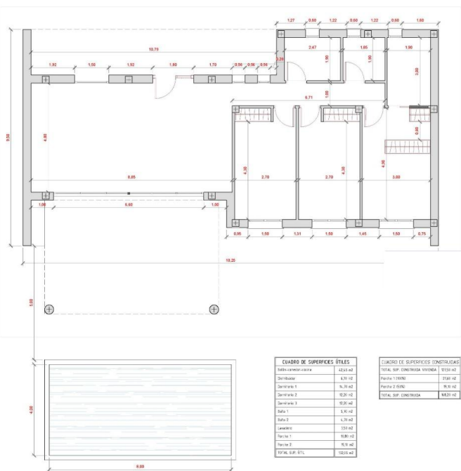
PLANTA COTAS E 1:50
