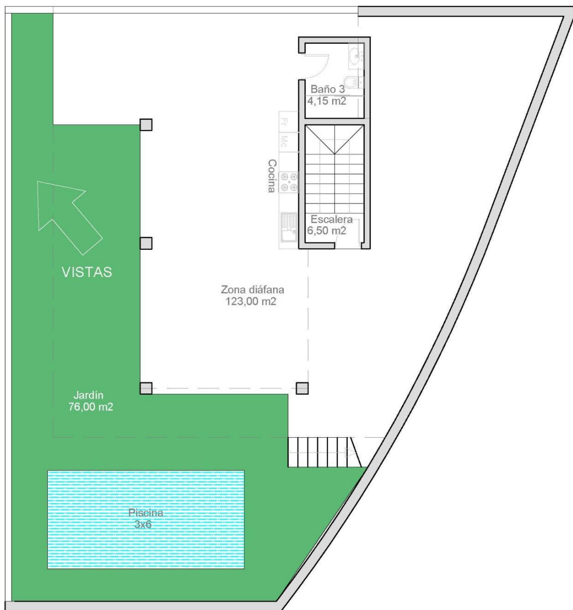
PLANTA BAJA
