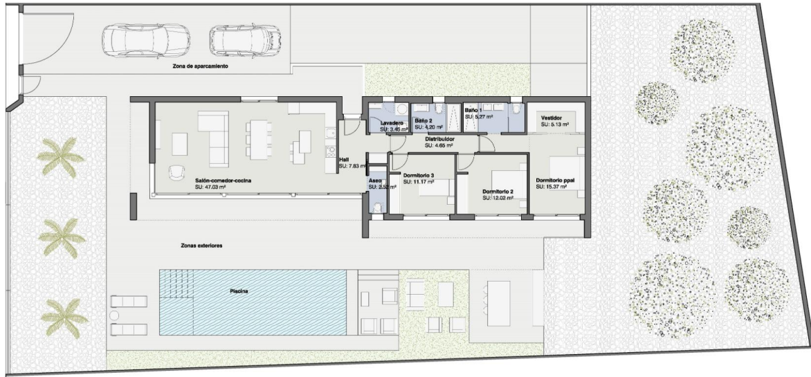
PLANTA BAJA
