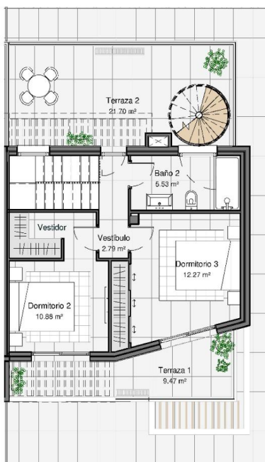
PLANTA PRIMERA
